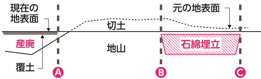
横断面図 No.15 (推定図)
